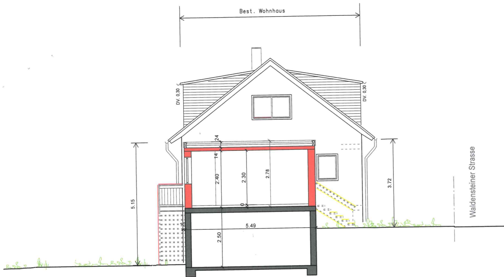
SCHNITT 1-1
