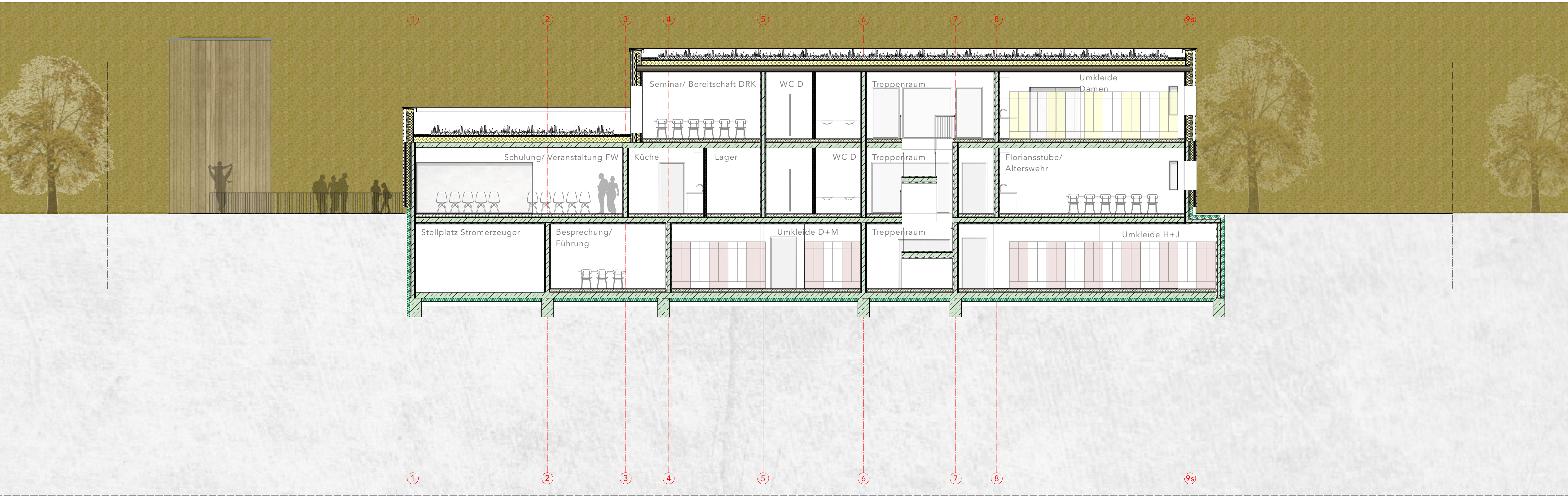
Schnitt B-B
