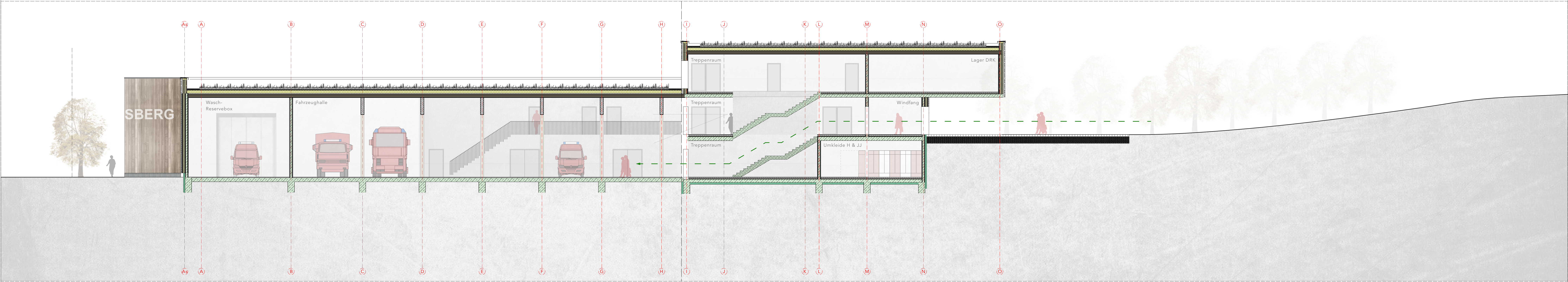
Schnitt AA
